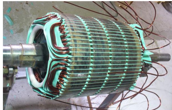
Dieser E-Motor stammt aus der Greiffenberger Motormühle, die in den 30er Jahren in Konkurrenz zur Erdholländermühle gebaut wurde. Durch PCK und EAB wurde er komplett restauriert und dient heute als Antrieb für den Mahlgang. 2
